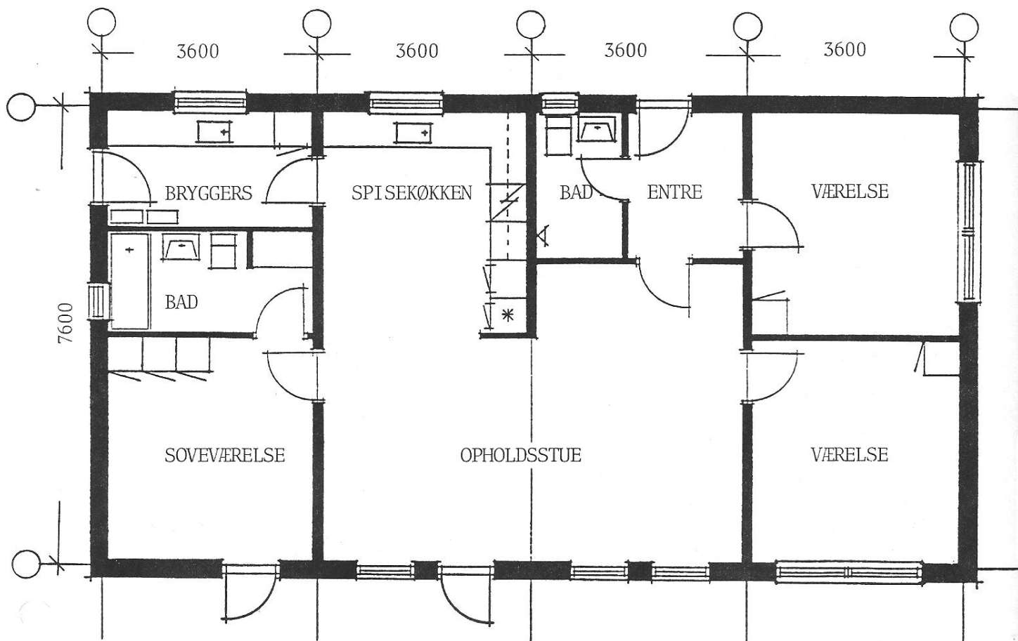
TYPE D GRUNDPLAN
